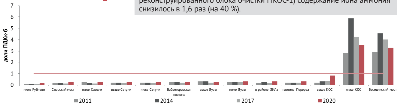
Рисунок 7. Иона аммония в створах Москвы-реки в 2011-2020 гг., доли ПДКк-б.
