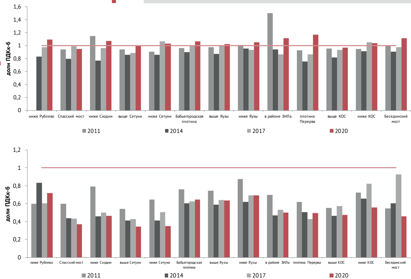
Рисунок 5. БПК5 в створах Москвы-реки в 2011-2020 гг., доли ПДКк-6.
