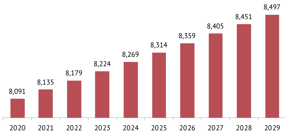
Рисунок 2. Прогноз образования ТКО в городе Москве с учетом отдельно собираемых ВМР до 2029 года (по данным Территориальных схемы).
