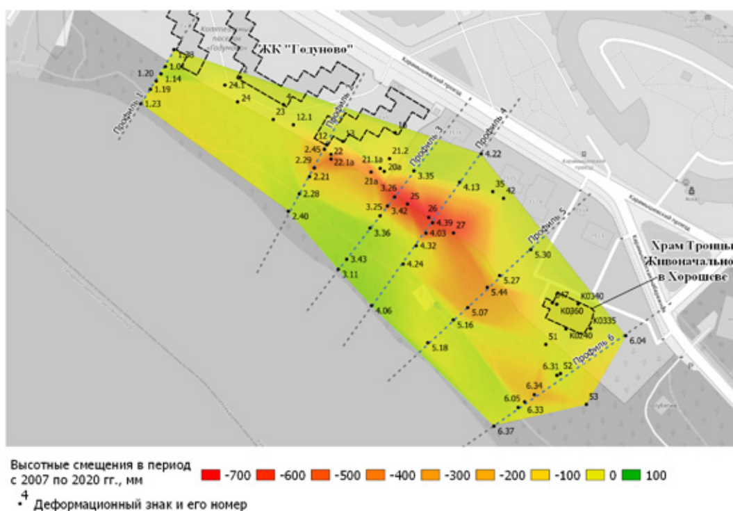
Рисунок 17 Карта вертикальных смещений приповерхностной зоны грунтов на оползневом участке Хорошево-1 за период 2007-2020 гг.
