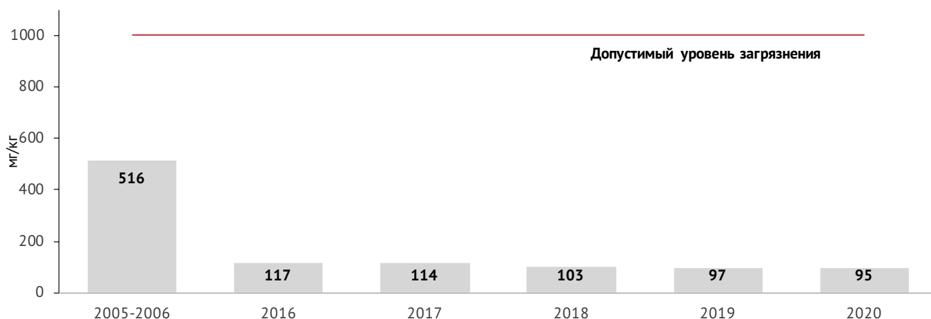
Рисунок 9. Динамика среднего содержания бенз(а)пирена в почве площадок постоянного наблюдения
