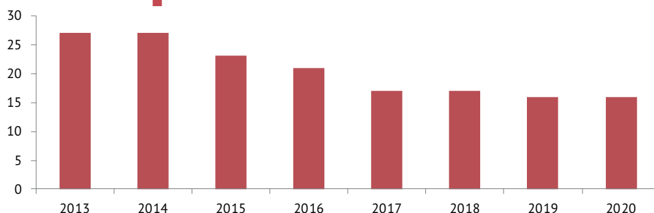
Рисунок 27. Количество выявленных карстово-суффозионных воронок, характеризующихся деформациями окружающей застройки
