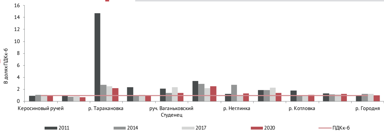
Рисунок 21. Взвешенные вещества в створах малых рек в 2011-2020 гг., доли ПДКк-б.
