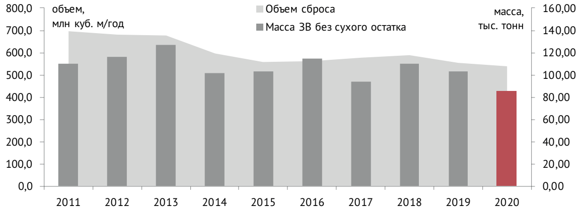
Рисунок 1. Объем сточных вод КОС и масса загрязняющих веществ КОС 2011-2020 гг.
