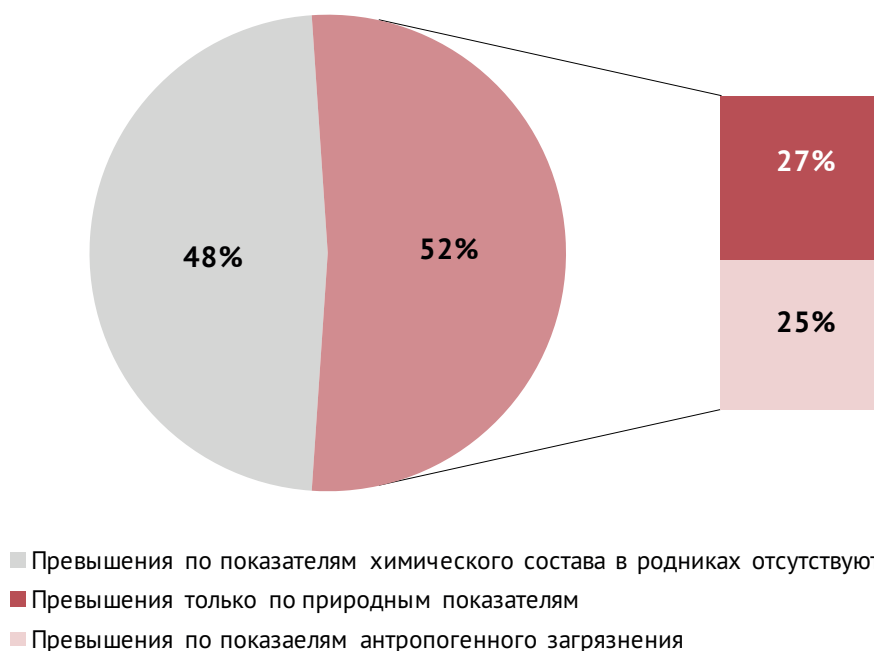
Рисунок 37. Соотношение долей родников с превышениями по показателям природного и антропогенного характера в 2020 году
