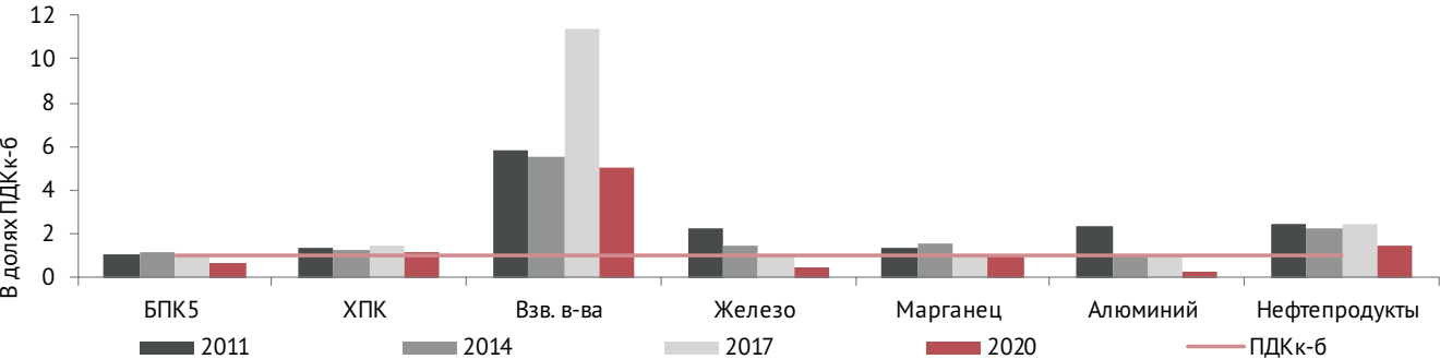
Рисунок 16. Среднегодовые концентрации основных анализируемых показателей в устье р. Сетунь в 2011-2020 гг., доли ПДКк-б.
