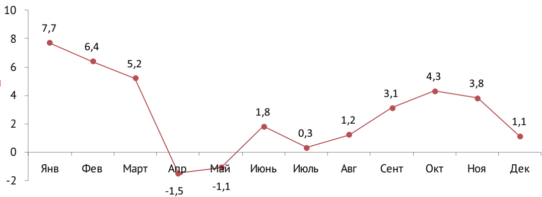
Рисунок 1. Отклонение (аномалии) средних месячных температур воздуха от нормы в 2020 году по данным наблюдений метеорологической станции Москва (ВДНХ)
