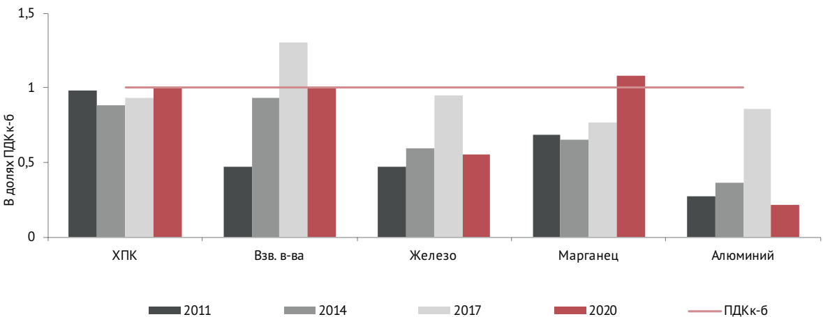
Рисунок 15. Среднегодовые концентрации основных анализируемых показателей в устье р. Сходни в 2011-2020 гг., доли ПДКк-б.
