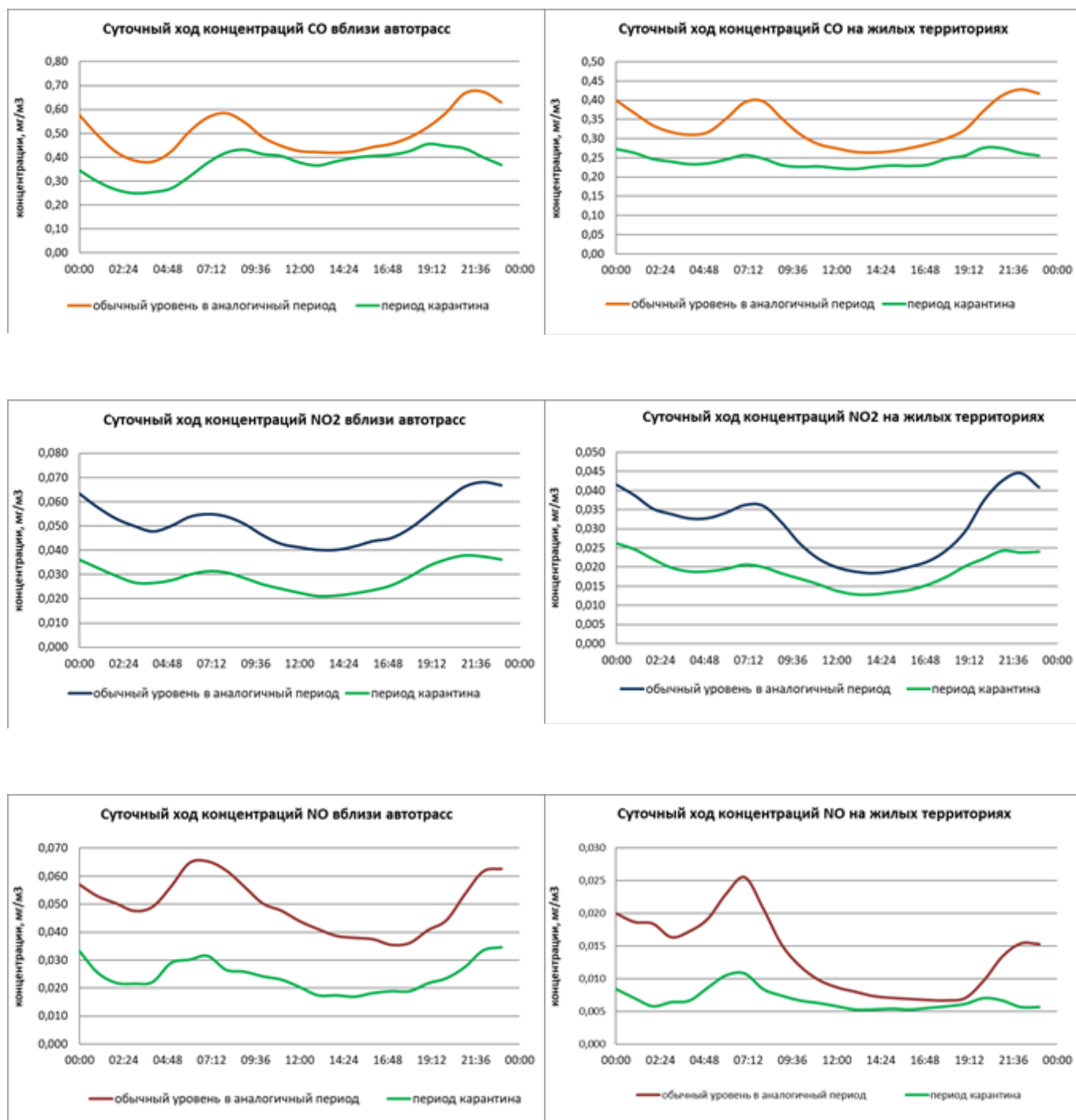
Рисунок 9. Суточный ход концентраций загрязняющих веществ в апреле 2020 года в период самоизоляции.
