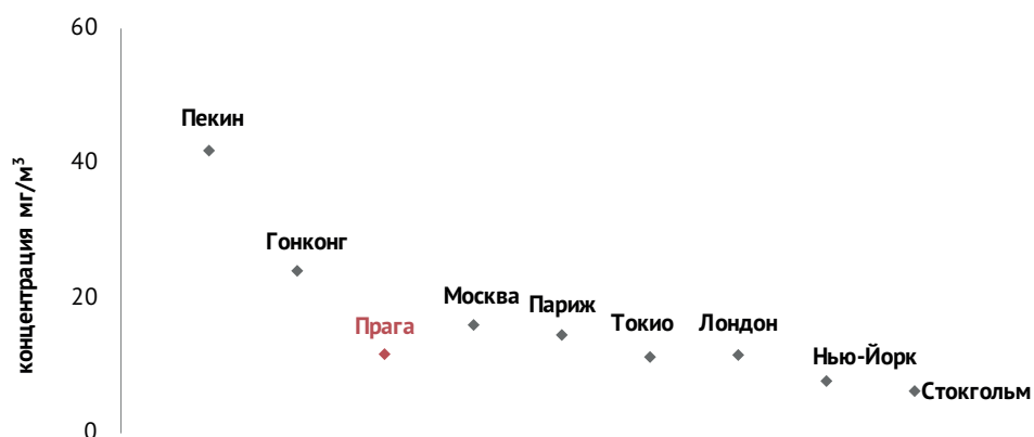
Рисунок 9. Среднегодовые концентрации PM 2,5 в атмосферном воздухе в 2019 году
