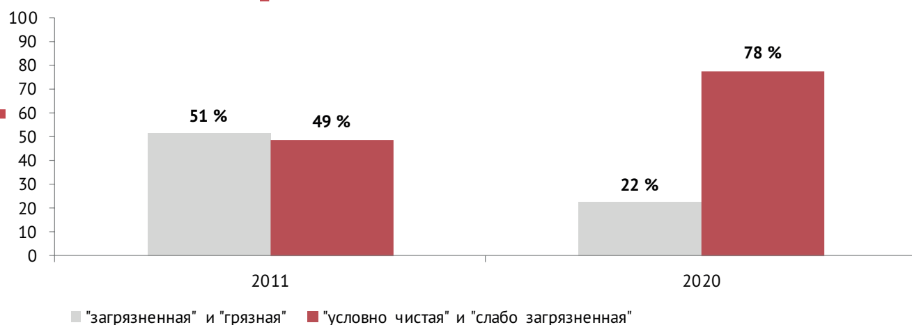
Рисунок 3. Динамика изменения состояния водотоков города Москвы в контрольных створах в 2011-2020 гг.
